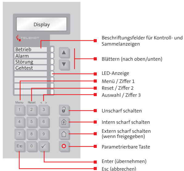
Aufbau BT 820
