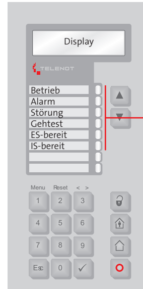
Bedienteil LED-Anzeige
